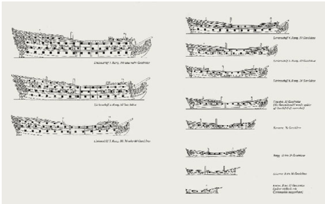
8 Im 17. Jahrhundert wurden mit Entwicklung der Kiellinientaktik die Kriegsschiffe nach ihrer Größe und der Anzahl ihrer Kanonen in Ränge eingeteilt.
